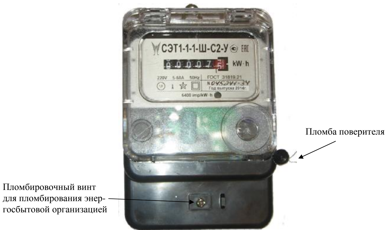
Рисунок 3 Фотография внешнего вида счетчиков СЭТ1 в универсальном корпусе для установки на поверхность или DIN-рейку («У»).
