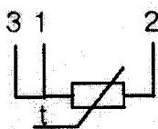
Схема 3 - трехпроводная
