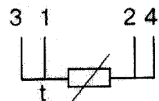
Схема 4 - четырёхпроводная
