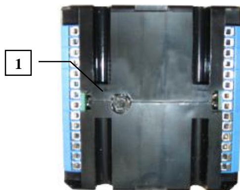
Рисунок 3 – Защита приборов Т-424 от несанкционированного вскрытия с помощью поверительного клейма
