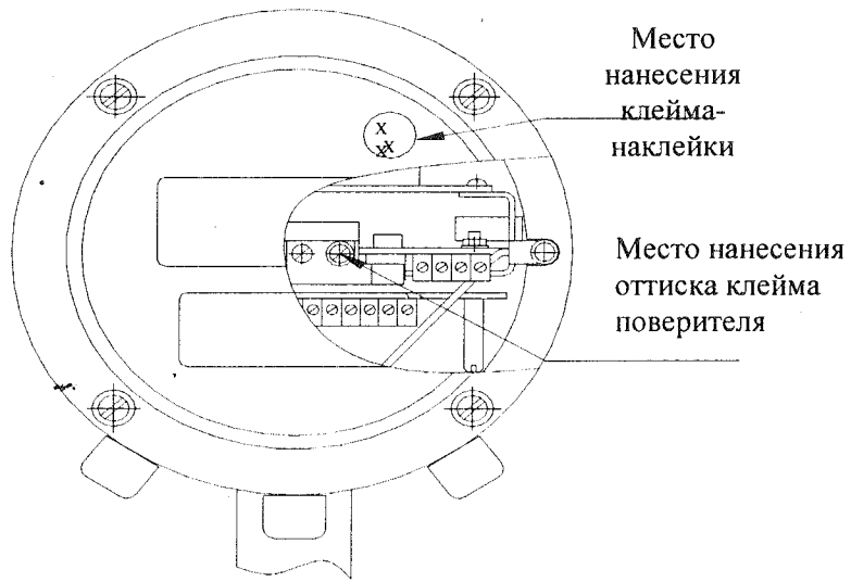
а) исполнение РСМ - 05.01
