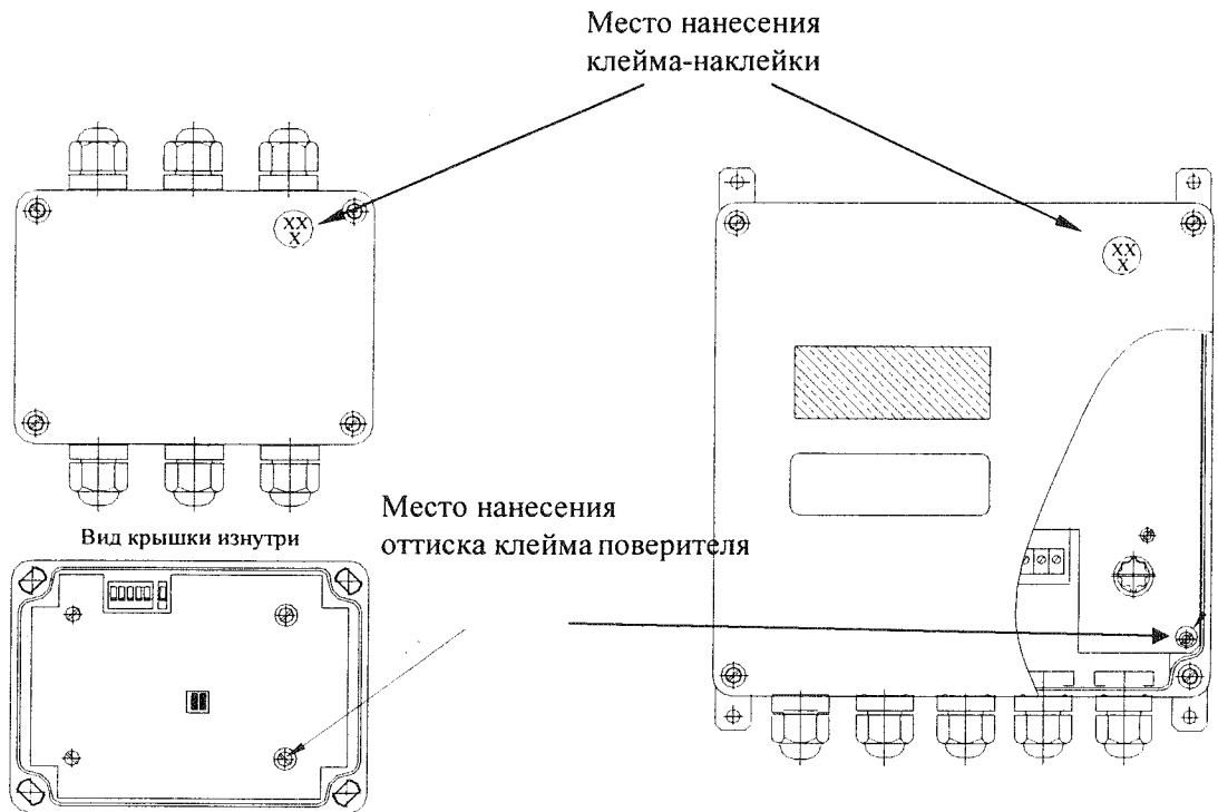
б) исполнение РСМ - 05.05, РСМ - 05.07
