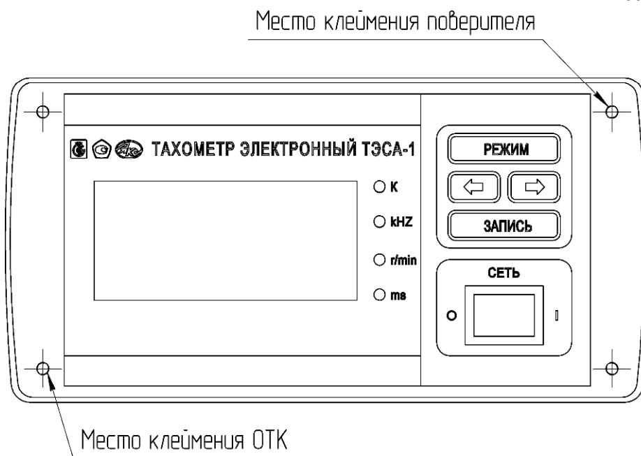
Рисунок 1- Вид на переднюю панель измерительного блока тахометра
