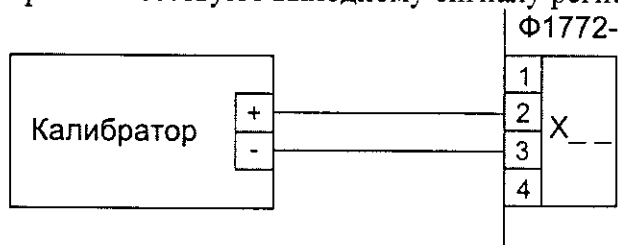
Рисунок 2 – Подключение входных сигналов постоянного напряжения, термопар и сигналов постоянного тока
