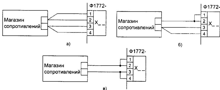
Рисунок 3 – Подключение входных сигналов сопротивления и термометров сопротивления: а) четырёхпроводная схема, б) трёхпроводная схема, в) двухпроводная сема
