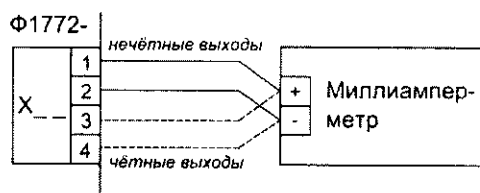
Рисунок 4 – Подключение выходных сигналов
