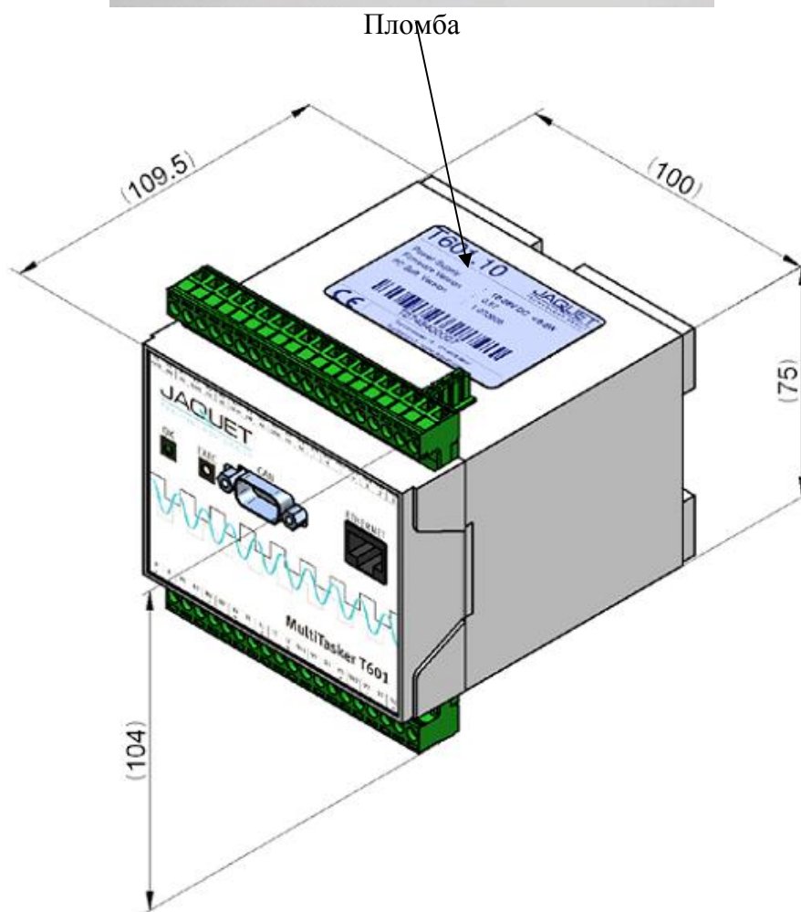
Рис. 3 Общий вид тахометра T600, схема пломбировки от несанкционированного доступа
