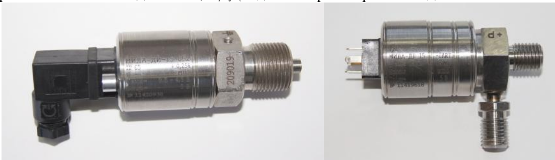
Рис. 1. Общий вид датчиков давления МИДА-15
