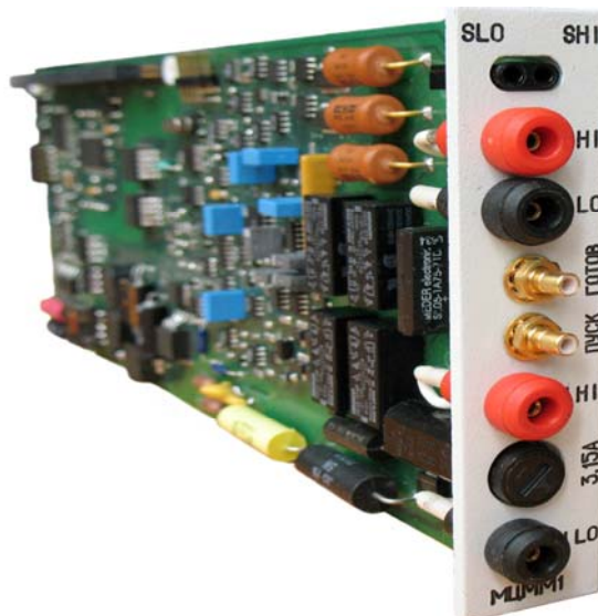
Рисунок 4 – Внешний вид мультиметра цифрового МЦММ1 UNC3.031.145
