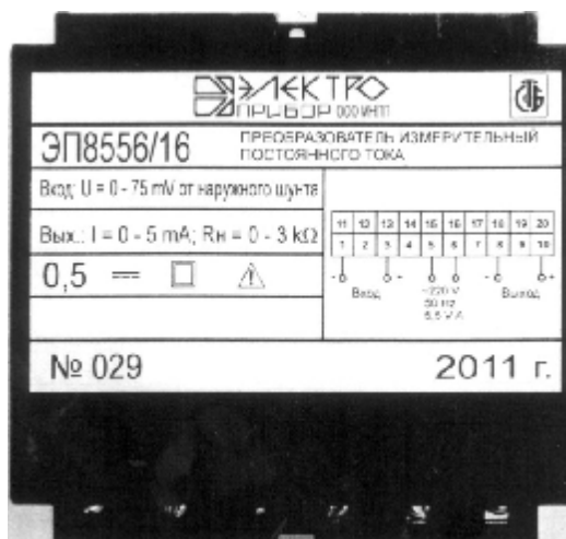
Рисунок 1 – Внешний вид преобразователя измерительного постоянного тока ЭП8556
