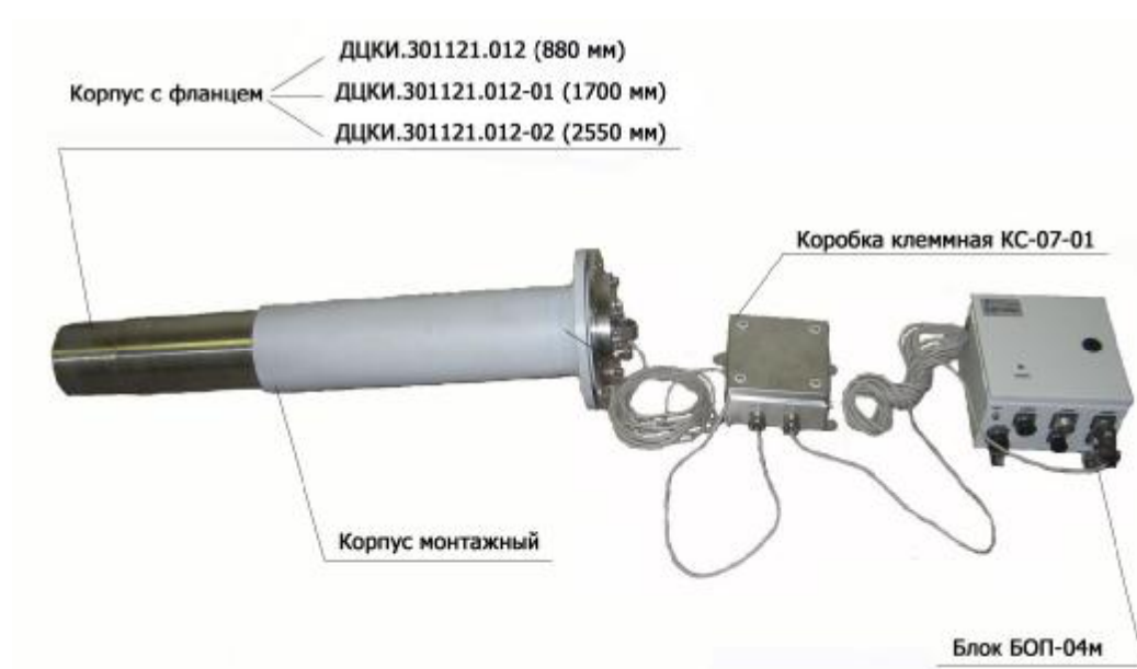
Рис. 2. Внешний вид установки радиометрической УДЖГ-42Р-07.
