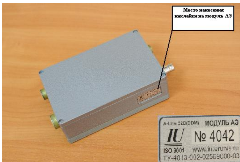
Рисунок 4 – Модуль АЭ
