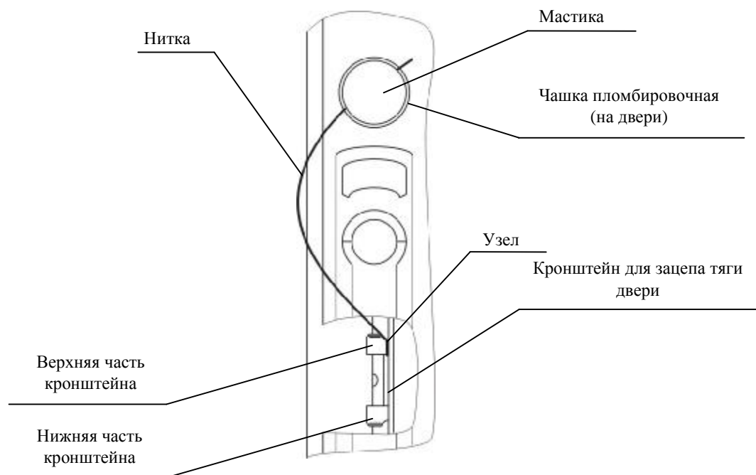
Рисунок 2 – Схема защиты от несанкционированного доступа
