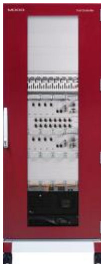
Рисунок 2 – Внешний вид аппаратуры для измерений механических воздействий и управления процессом проведения испытаний изделий машиностроения модели Aerospace Test Controller
