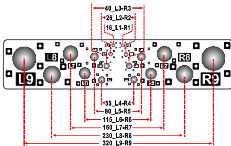
Рисунок 2 - Схема обозначения измеряемых параметров
