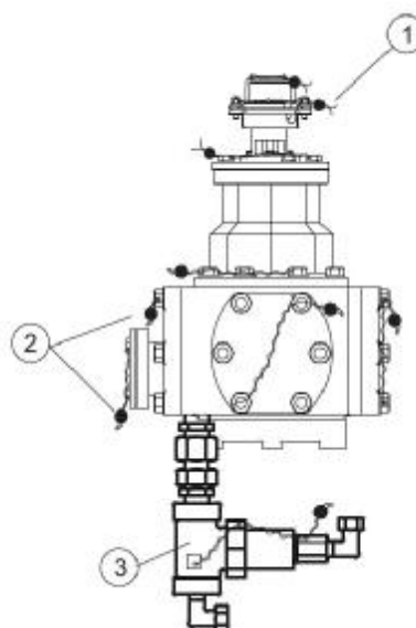
Р и с у н о к 3 – Схема пломбировки «YGM» фирмы «Yenen Engineering AS», Турция.
