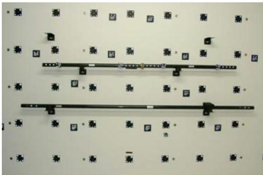
Рисунок 1 - Общий вид мер Scale Bar, закрепленных на стене.
