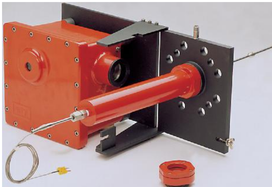
Рисунок 1 - Общий вид пирометров инфракрасных Pulsar II М7000 и Pulsar III М7000
