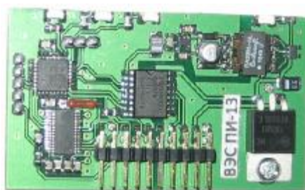
Рисунок 9. Модификация ВЭС ПИ - 13
