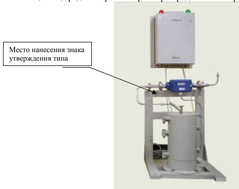
Рис. 1. Общий вид радиометра-спектрометра МАГ-031 (МАГ-031-01)
