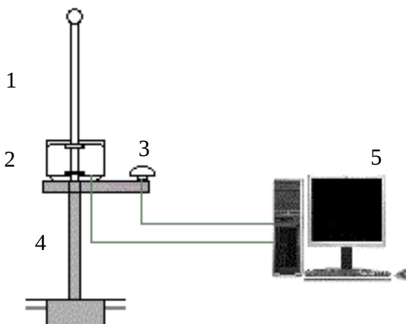
Рис.1 Общий вид регистраторов грозовой опасности «Алвес 7.04»: 1 – антенна регистрации электрической компоненты ЭМИ; 2 – защитный корпус антенного модуля; 3 - антенна GPS приемника; 4 - несущая стойка; 5 - рабочее место оператора.
