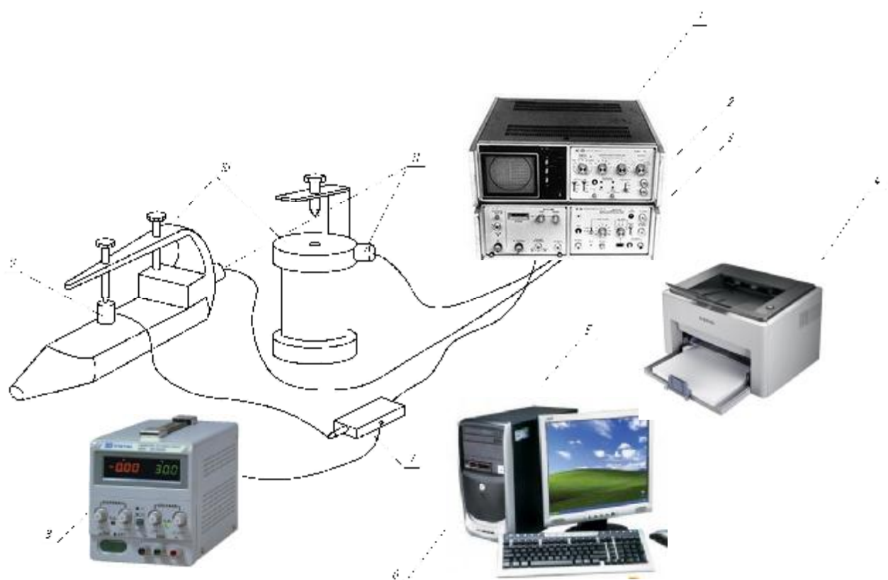
Рисунок 1 - Состав установки AP8004
