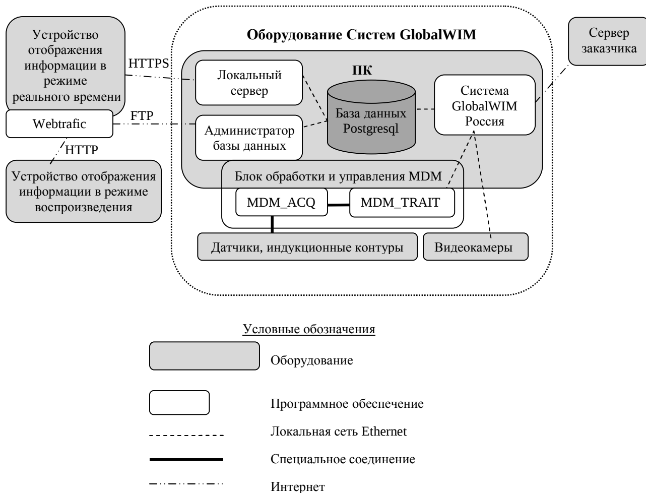
Рисунок 3 – Структура ПО Систем GlobalWIM
