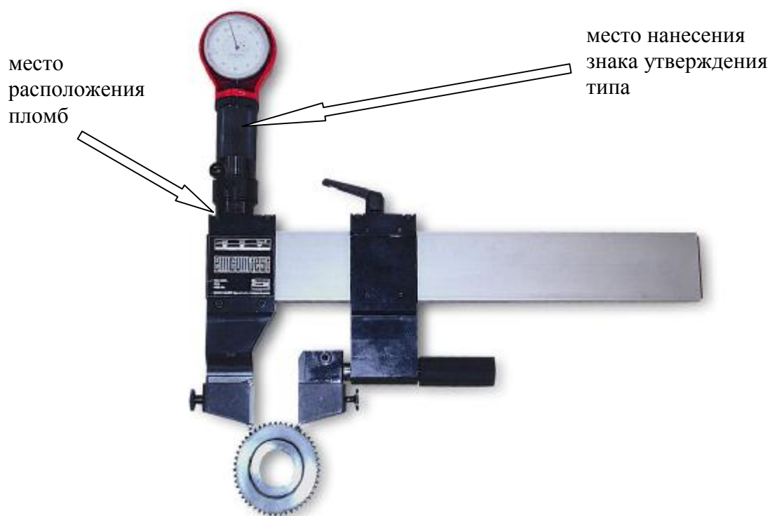
Рисунок 1 – Внешний вид твердомеров
