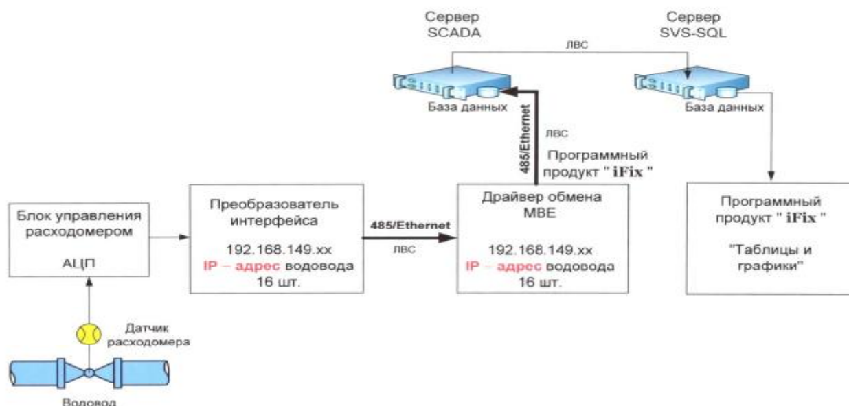
Рисунок 1 - Структурная схема АСДКУ
