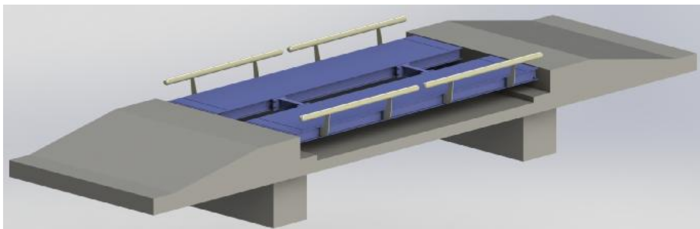
Рисунок 1 – Общий вид ГПУ весов автомобильных M8200Б
