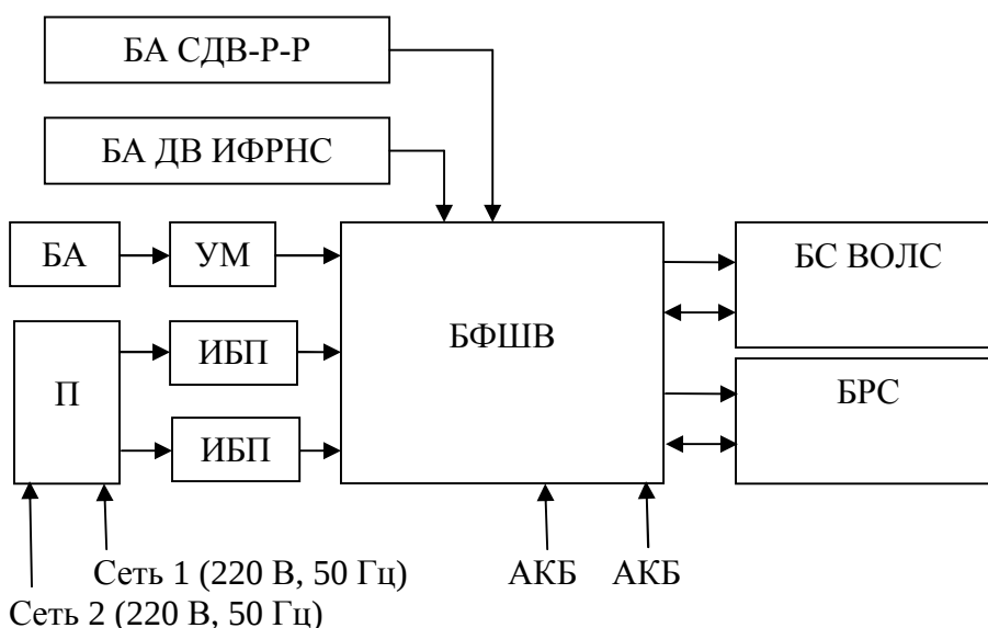
Рисунок 1 – Структурная схема ЦП-СЕВ
