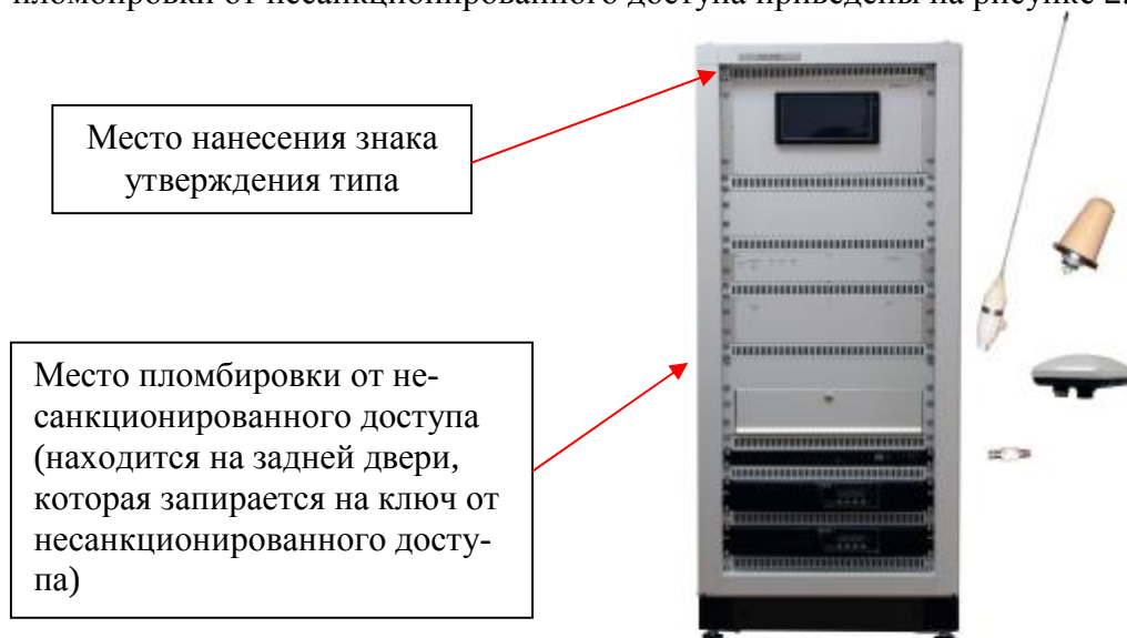
Рисунок 2 - Внешний вид ЦП-СЕВ и схема пломбировки
