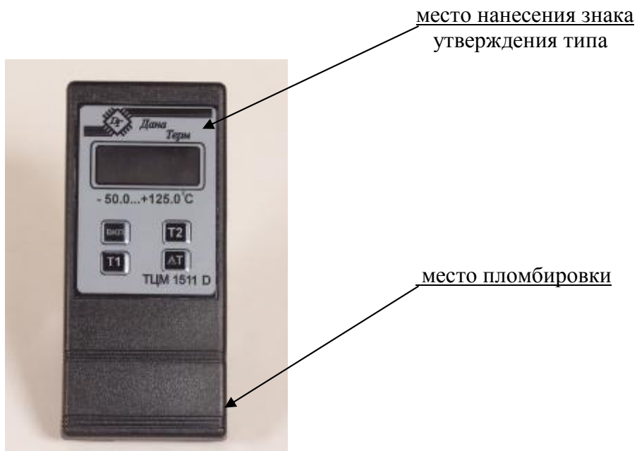
Рисунок 2 - Внешний вид TCМ 1511
