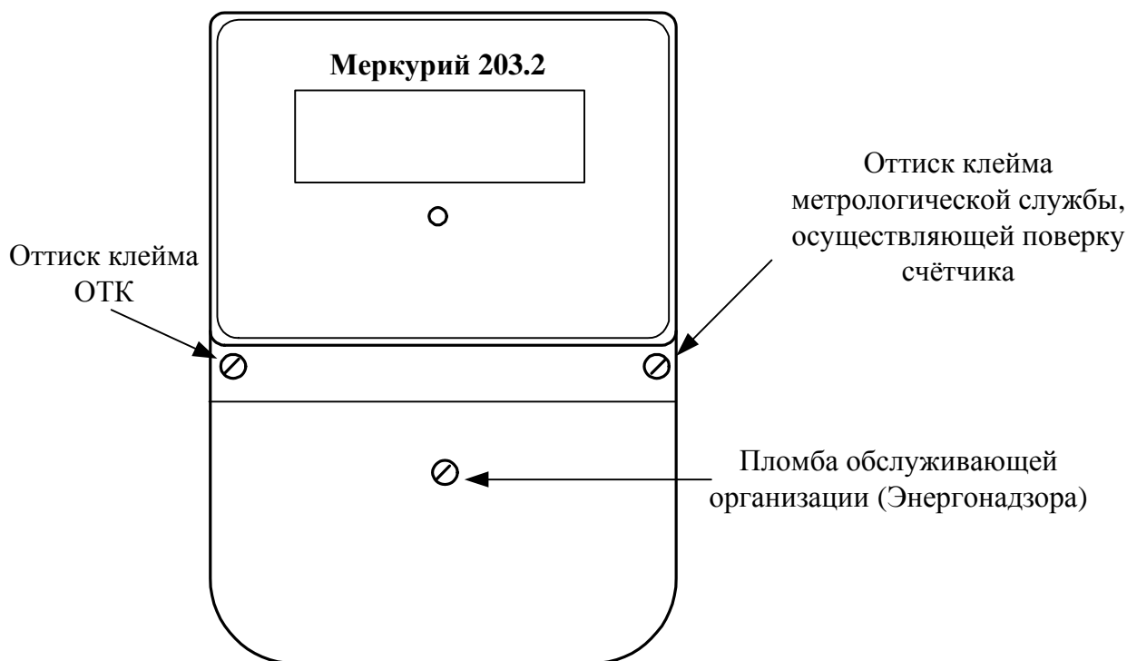
Рисунок 4 - Схема пломбирования счётчика
