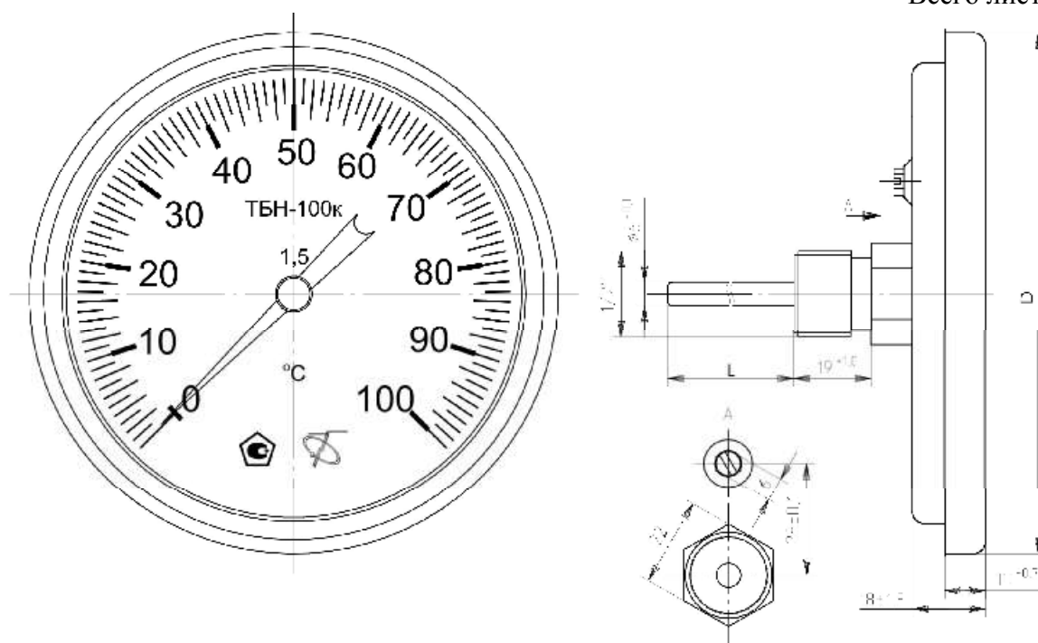
Рисунок 2 - термометр ТБН.
