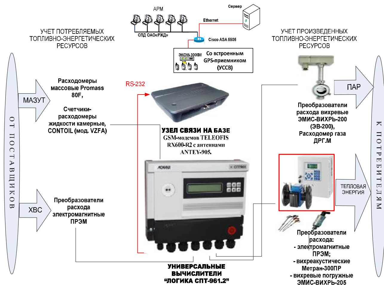
Рисунок 1 - Структурно-функциональная схема АСКУ ТЭР
