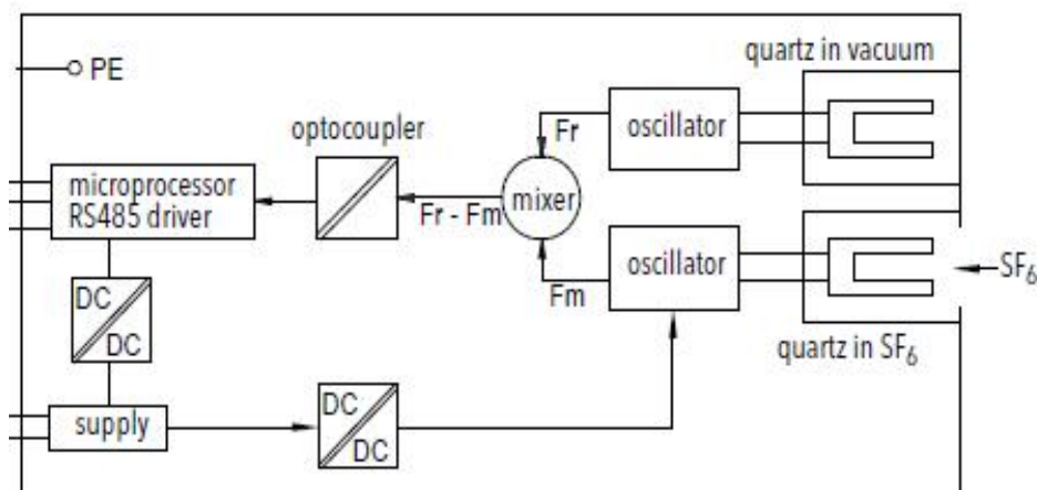
Рис. 1. Принципиальная схема плотмера элегаза серии 879X.
