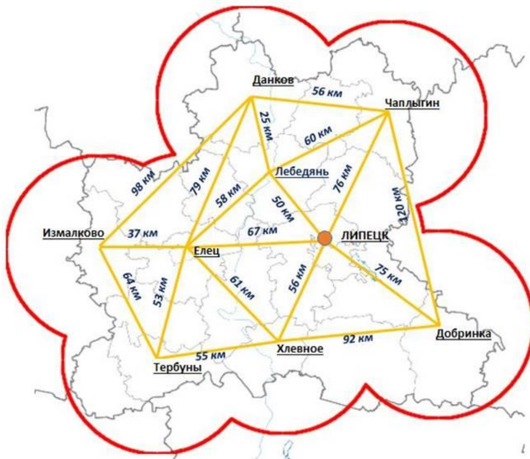
Рисунок 1 – Схема расположения референчных станций.
