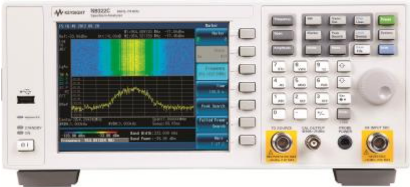
Рисунок 1 – Фотография общего вида анализаторов
