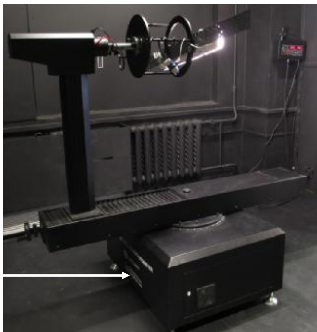
Рисунок 1 - Общий вид гониофотометра LSG-1800B, место его маркировки и пломбирования
