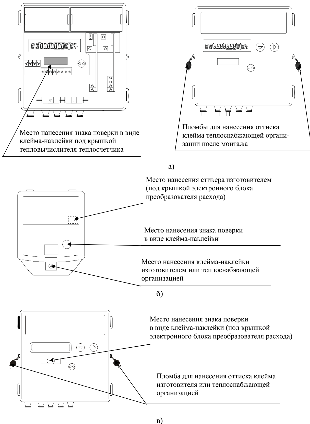
Рисунок 2 – Место клеймения после поверки, а) тепловычислителя теплосчетчика; б) преобразователя расхода ультразвукового «СТРУМЕНЬ» T150 исполнение без дисплея; в) преобразователя расхода ультразвукового «СТРУМЕНЬ» T150 исполнение с дисплеем
