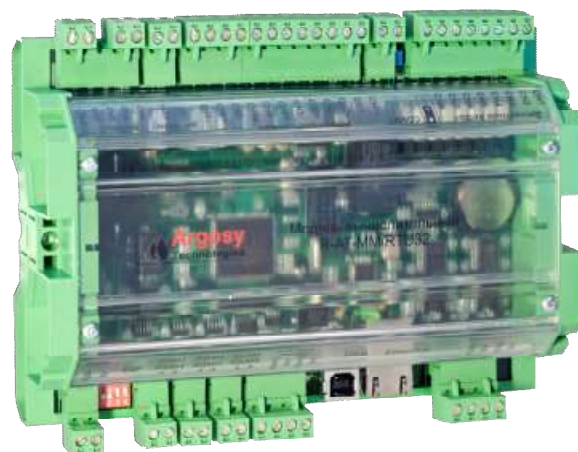
Рисунок 10 – модуль вычислительный (R-AT-MM/RTU32)
