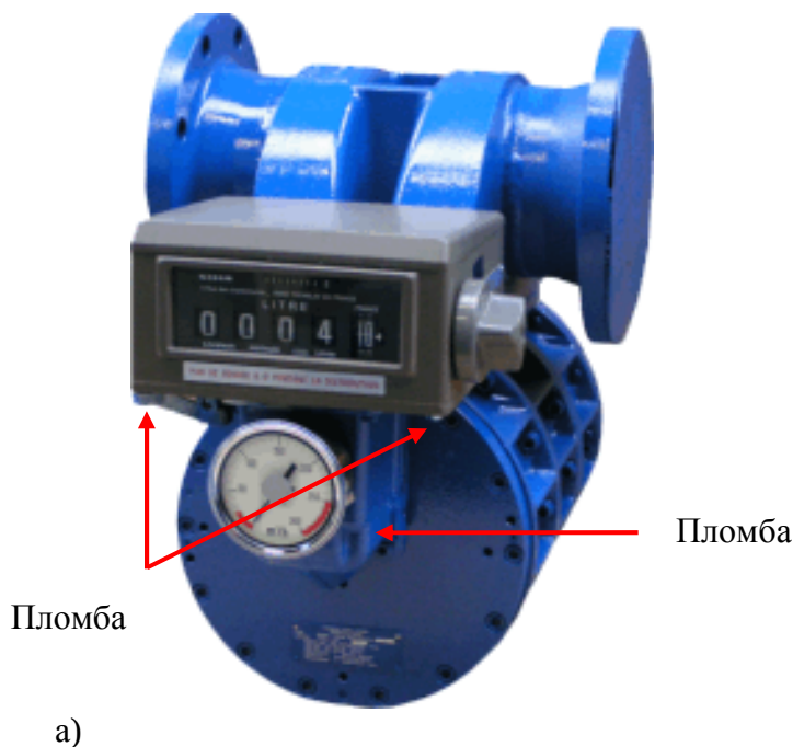
Рисунок 1 - Общий вид счётчиков нефтепродуктов ZC 17 80/80, ZC 17 80/150
