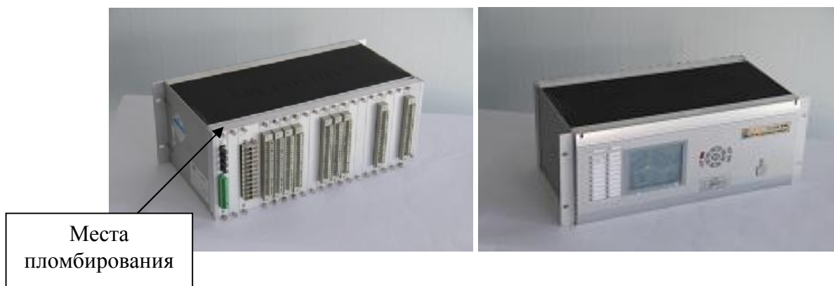
Рисунок 1б – Внешний вид устройства в корпусе «1» с дисплеем
