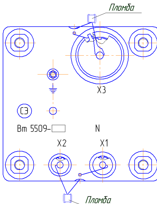
Рисунок 3 - Схема пломбировки от несанкционированного доступа
