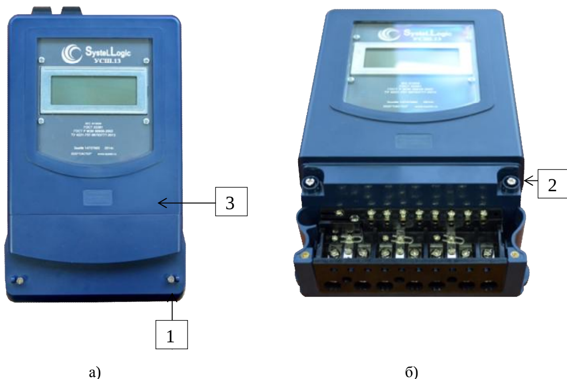
а) б) Рисунок 1 - Внешний вид модификаций УСШ а) в сборе; б) с отсоединенной нижней крышкой. 1. место пломбирования эксплуатирующей организацией; 2. место пломбирования на заводе изготовителе; 3. место нанесения знака поверки.
