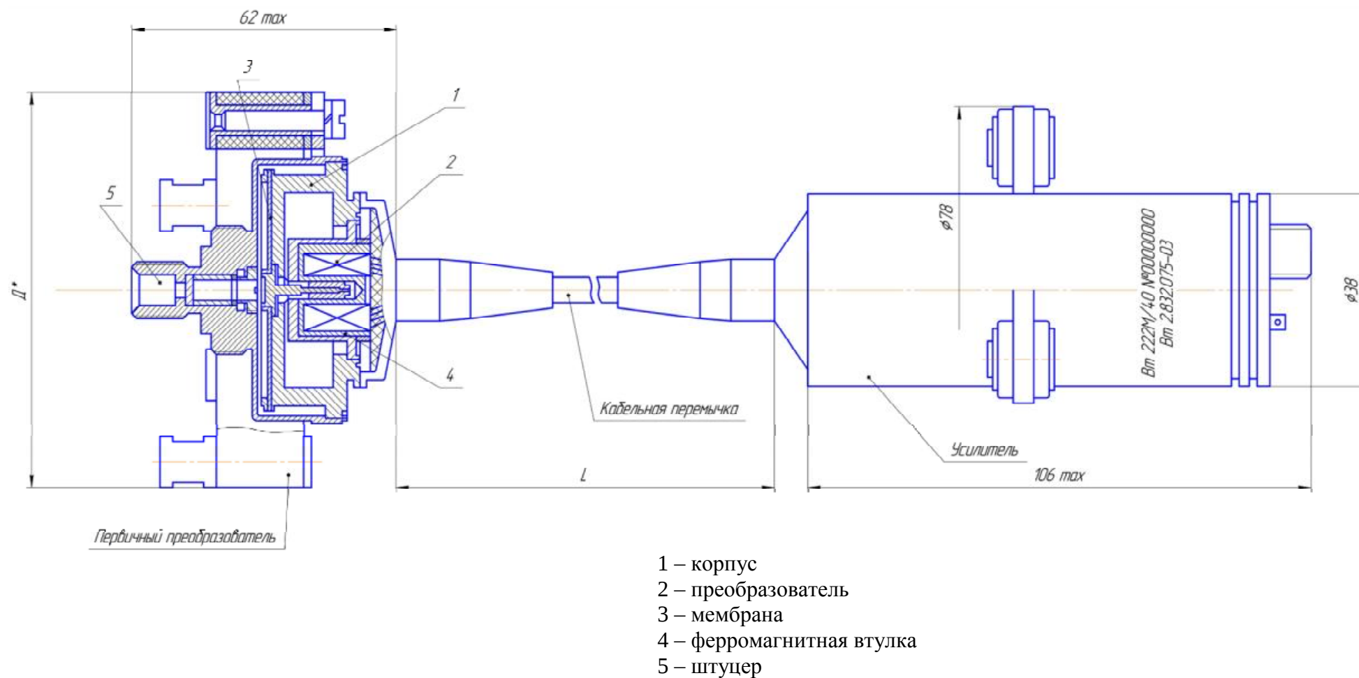
Рисунок 1 – Общий вид датчика Vm 222M
