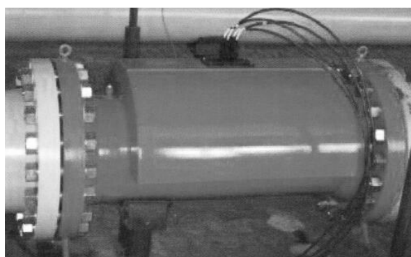
а) Внешний вид калиброванной измерительной трубы с датчиками, закрытыми кожухом
