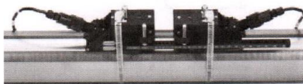
б) Внешний вид датчиков с монтажными рамами открытого типа
