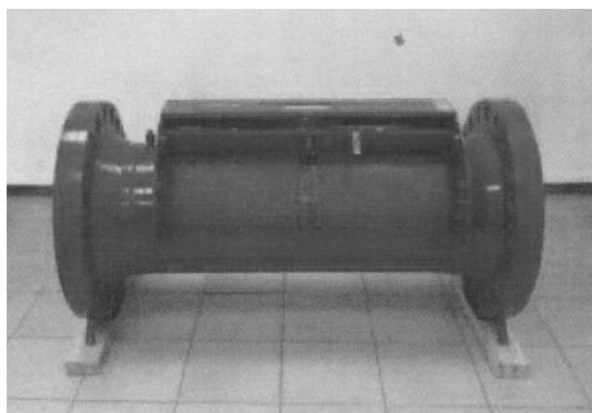
а) Внешний вид калиброванной измерительной трубы без датчиков
