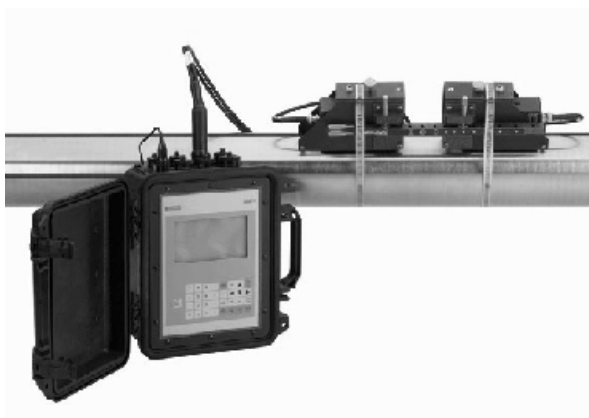
в) Внешний вид портативного вычислителя расходомера ГКС FUX1010
