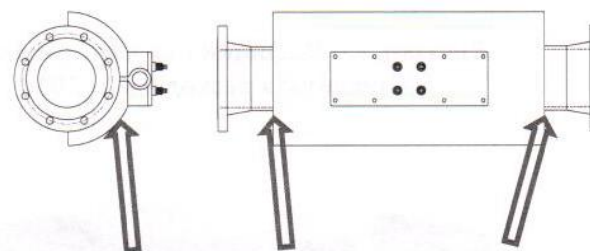
б) Схема нанесения пломб и знака поверки на калиброванную измерительную трубу с датчиками
