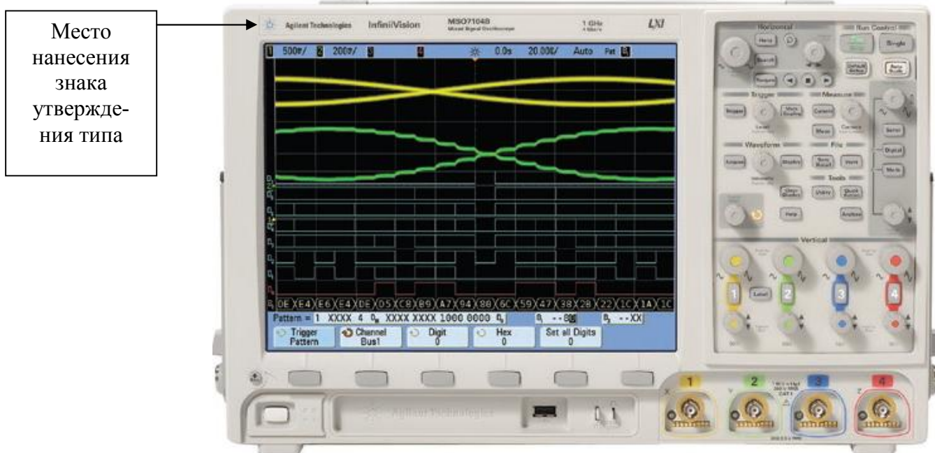
Рисунок 1 - Внешний вид одной из моделей осциллографа
