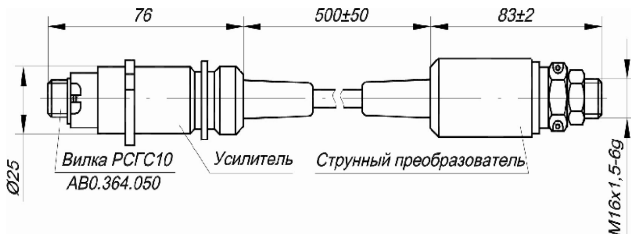
Рисунок 2 – Габаритные и установочные размеры датчика
