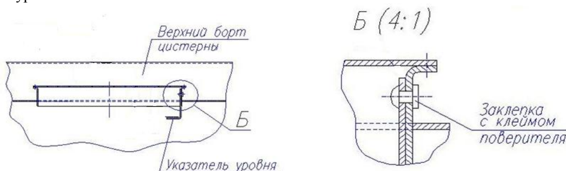
Рисунок 1 - Обозначение места для нанесения знака поверки
