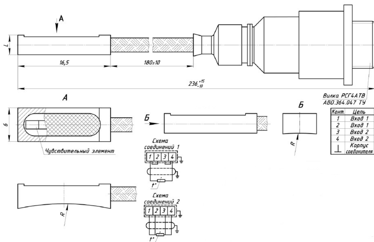
Рисунок 1 – Общий вид термопреобразователя
