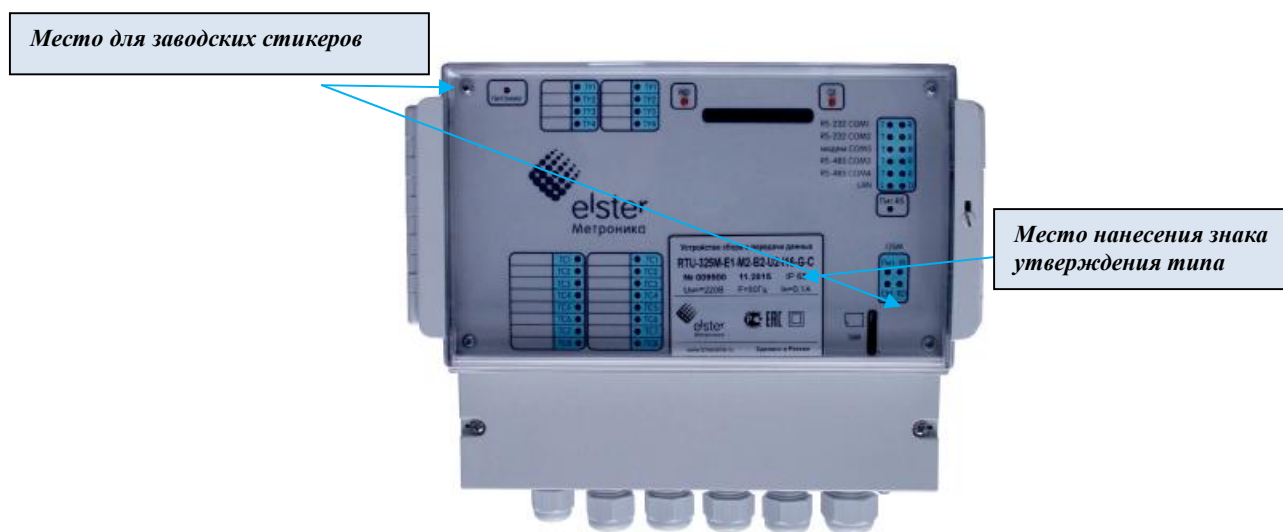
Рисунок 1 – Внешний вид УСПД RTU-325M
