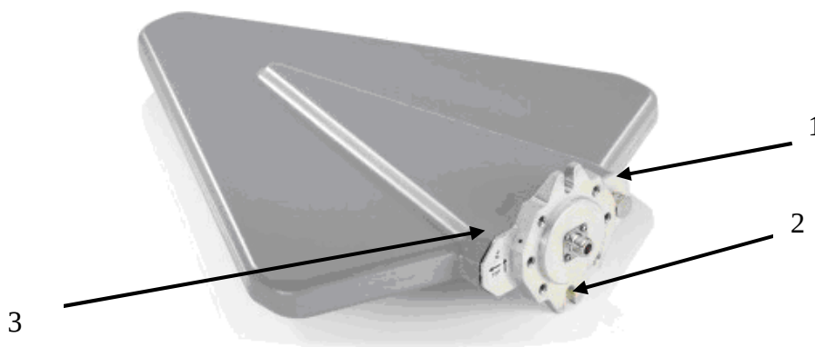
Рисунок 1 - Фотография общего вида антенн логопериодических R&S HL040E
