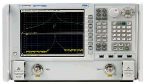
Рисунок 4 – Внешний вид векторного анализатора цепей
